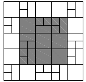
(D) 3 piece 7x7 - 22% 7x14 - 22% 14x14 - 56% Laying Ratio: 8:4:5
